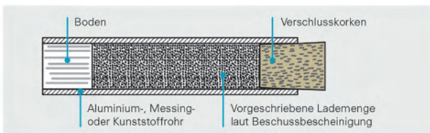
Abb. 43: Dosierung der Pulvermenge für einen Schuss (abgepackte Einzelladung)
